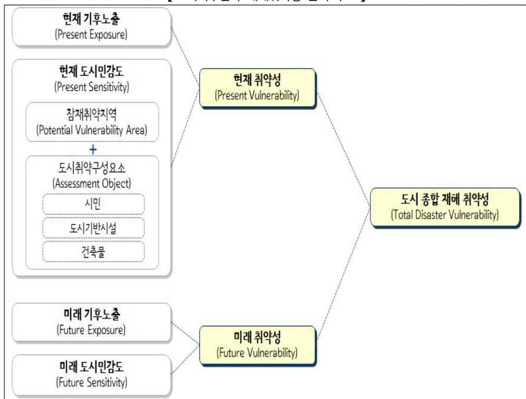
【 도시기후변화 재해취약성 분석 구조 】
