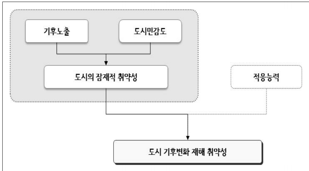
【도시기후변화 재해취약성 분석 개념】
